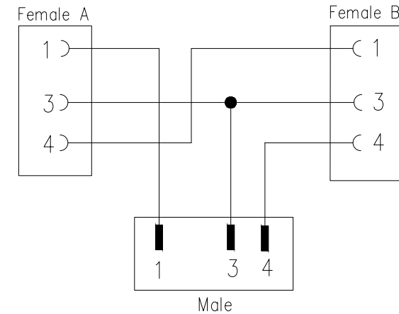
接线图: Circuit Diagram:
